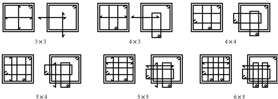
图 1-2 常见复合箍筋类型图
