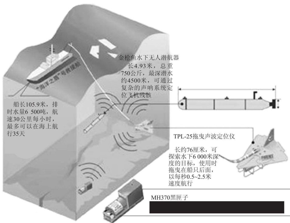
图 1-1 “金枪鱼牌”飞机黑匣子搜索仪工作示意图
