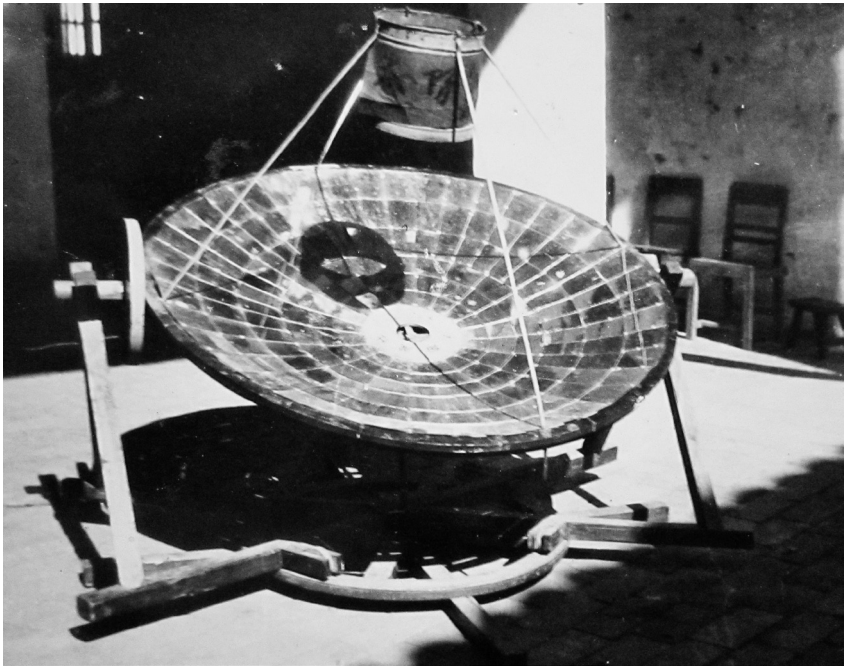
县商业局干部仿制成功的太阳灶
