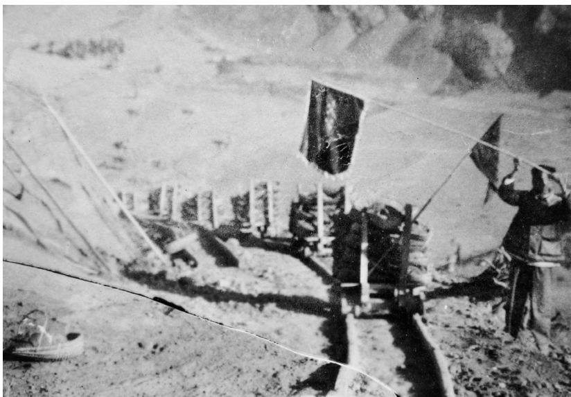
县农林局干部仿制成功的自动化有轨木车，在 200 米的山坡每分钟可运土一次，比人力搬运提高了 60 倍
