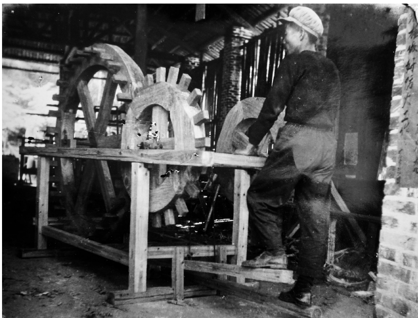
农生站干部研制成功的红薯工作母机，日可加工红薯 30000 斤
