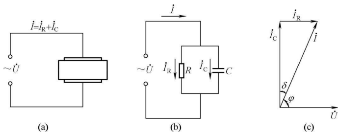
图 1-1 绝缘在交流电压作用下的等值电路和相量图
