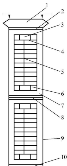
图 1-3 气外冷电机定子绕组槽部绝缘结构
