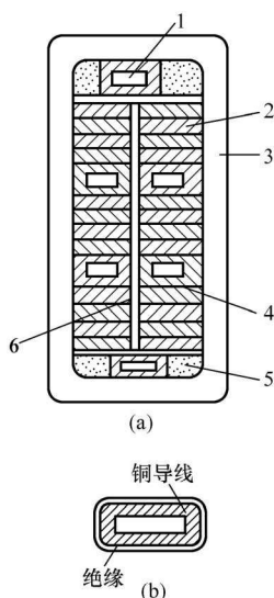
图 1-4 水内冷电机定子绕组槽部绝缘结构
