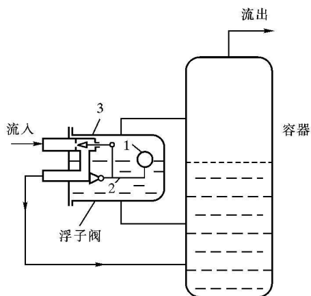
图 1.3 液位的自动控制系统 1—浮子;2—杠杆机构;3—阀件
