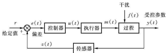
图 1.4 自动控制系统方框图
