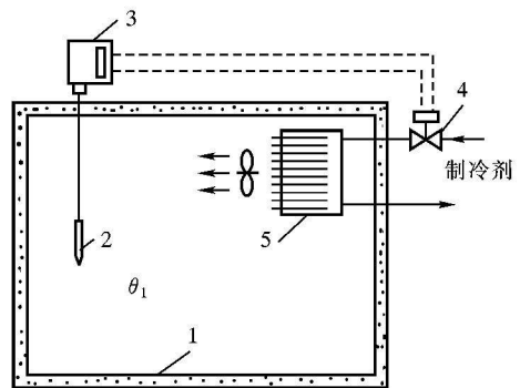
图 1.2 库房温度自动控制系统
