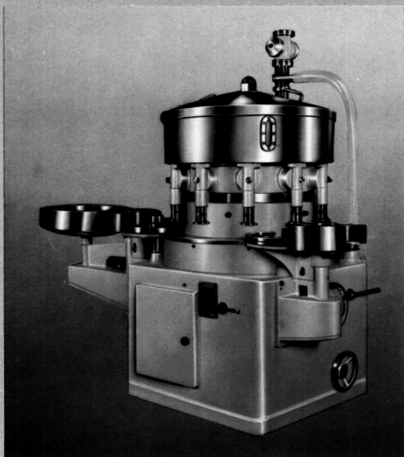
Z6 — 10 自动酱汁灌装机
