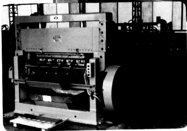
SMD—002 自动 波形剪板机
