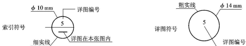
图 0-1 被索引的详图在同一张图纸内
