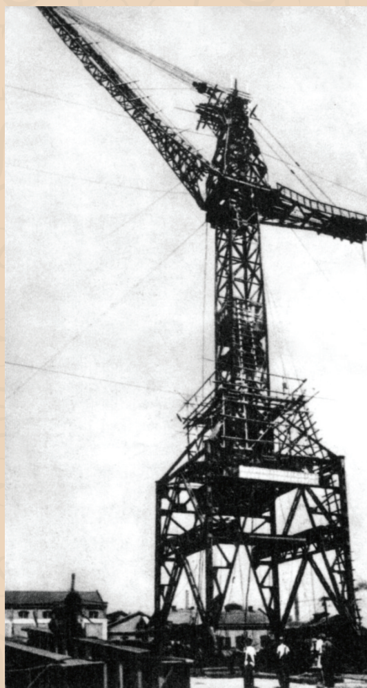
1955年10月，沈阳桥梁厂试制成功中国第一台大型起重设备——25吨塔式起重机。该机自重280吨，高54米，相当于15层楼房，最高扬臂72米，最大起重半径35米，最大提升高度64米，可360度旋转
