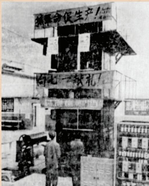
1967年8月4日，中国第一台立式红外线硫化设备在沈阳第四橡胶厂试制成功
