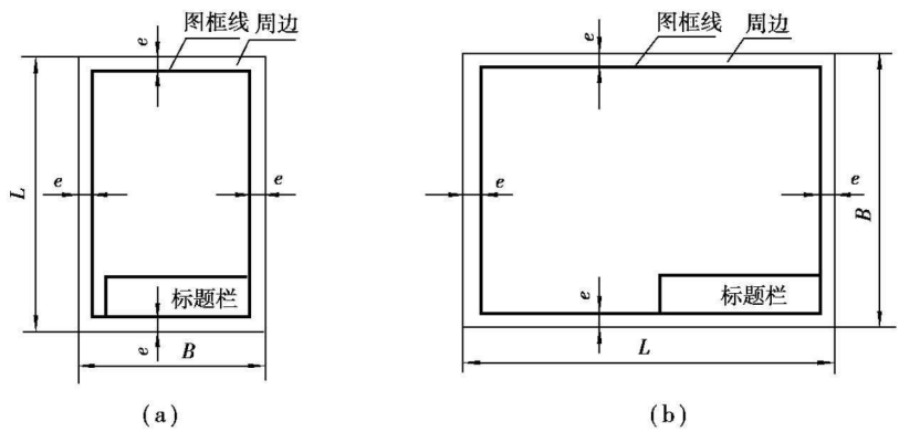
图 1-3 图框格式
