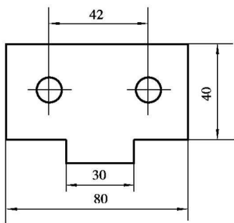
图 1-11 尺寸线
