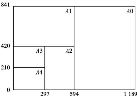
图 1-1 图纸幅面尺寸关系
