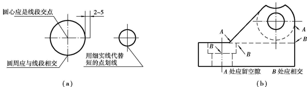
图 1-8 图线画法举例
