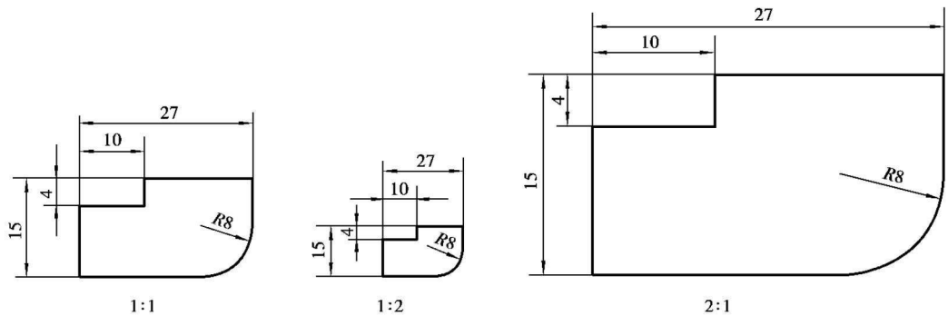
图 1-5 机件用不同比例画出的图形
