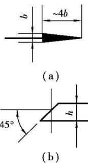
图 1-12 尺寸终端形式
