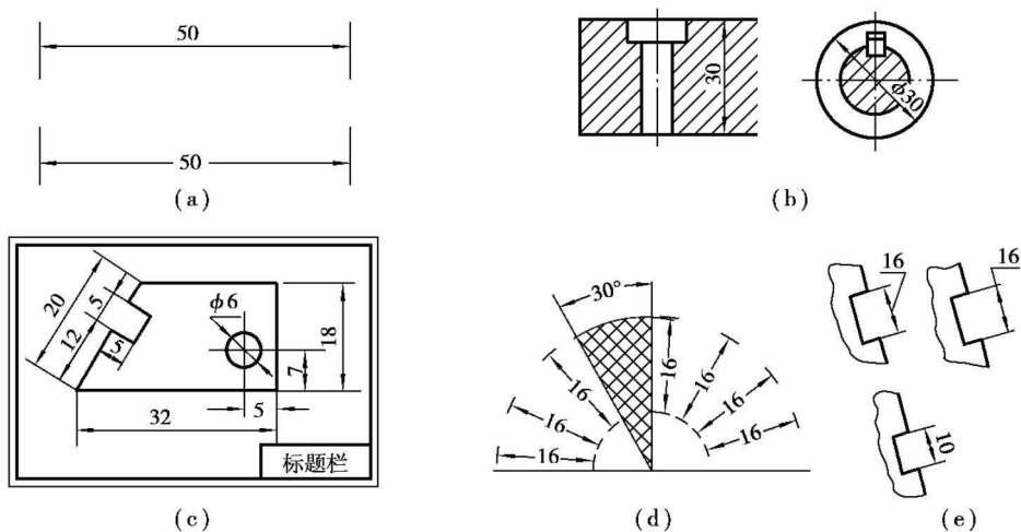
图 1-13 注写尺寸数字的方向及规定
