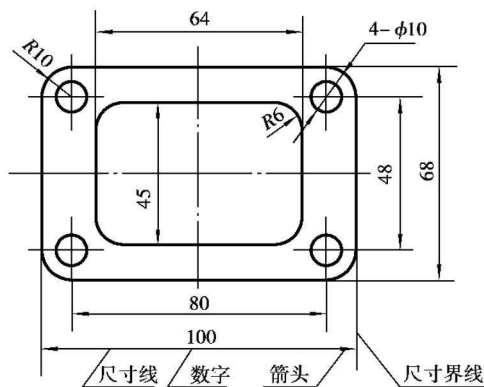
图 1-9 尺寸的组成及标注示例
