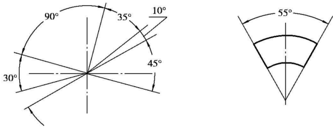
图 1-15 角度尺寸的注法
