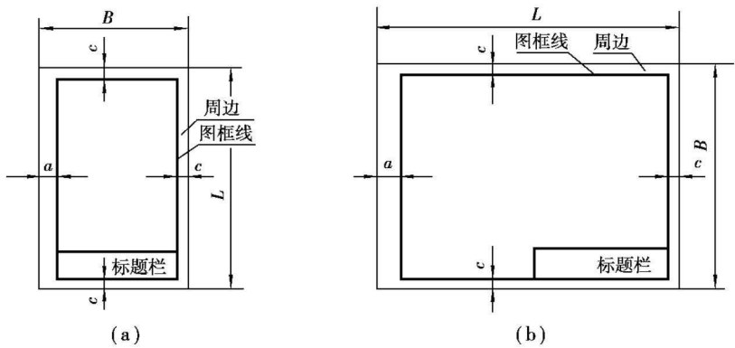
图 1-2 图框格式
