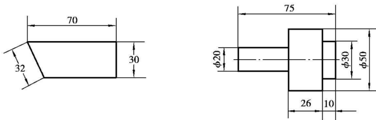
图 1-14 尺寸数字水平注法
