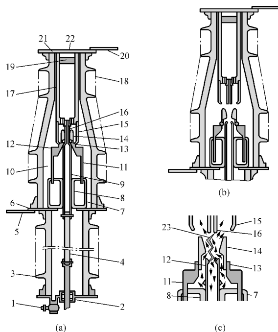
图 1-2 自能式 SF 6 断路器灭弧室结构及灭弧原理图 (变开距)
