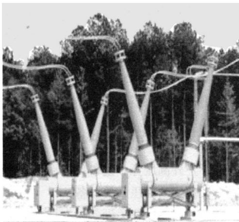
图 1-6 罐式断路器 (LW13-550)
