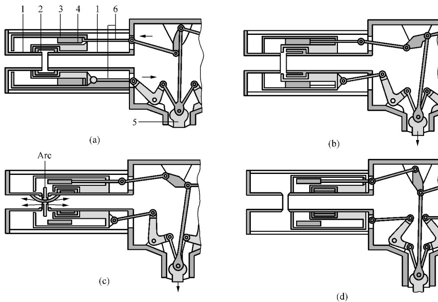
图 1-4 定开距灭弧室开断过程示意图
