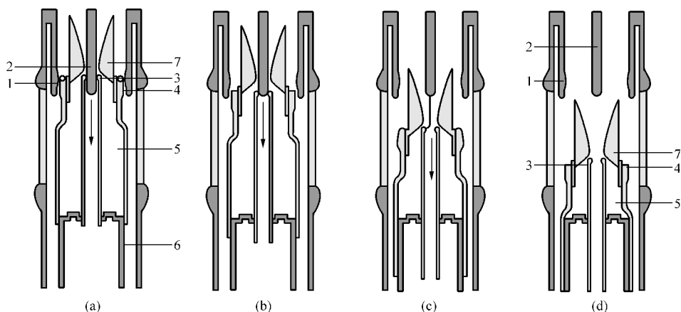
图 1-3 变开距灭弧室开断过程示意图
