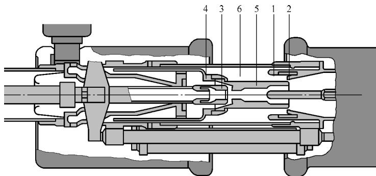
图 1-1 ABB 公司 GIS 用 SF 6 断路器灭弧室机构图
