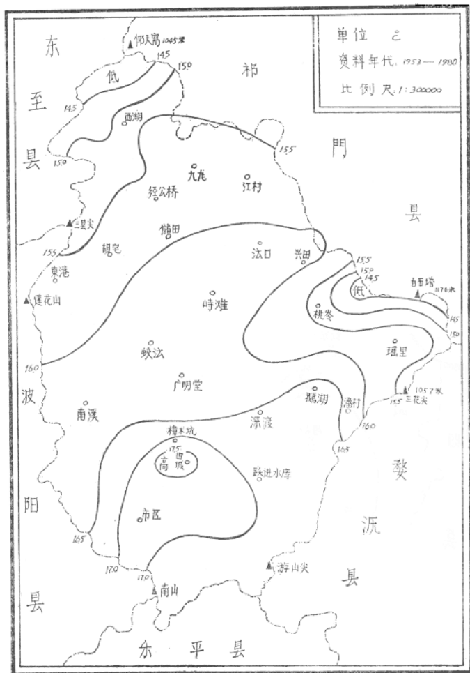
景德镇市各地年平均气温分布图 (1953—1980年)
