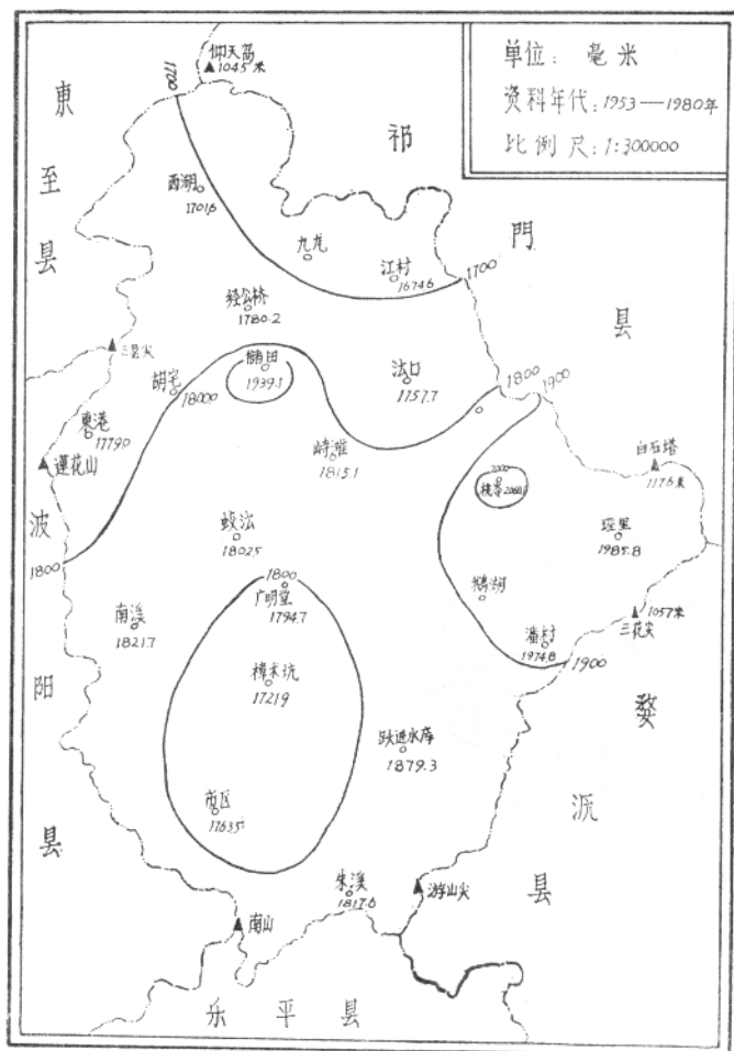
景德镇市各地多年平均年降水量分布图 (1953 — 1980年)
