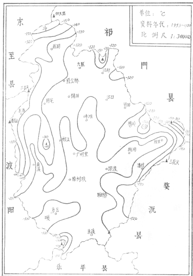
景德镇市各地极端最低气温分布图 (1953—1980年)
