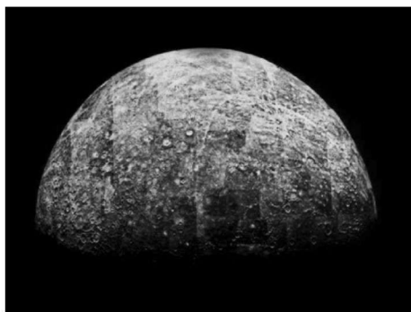
水星表面
