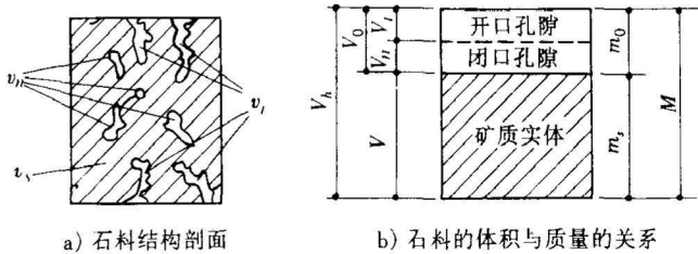
图 1-1 石料的体积与质量关系示意图
