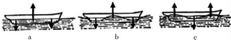
图1-1-3 浮力和重力引起的纵向弯曲
