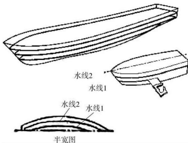
图 1-1-15 水线面与半宽水线图
