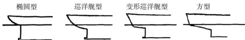
图 1-1-11 艏部形状
