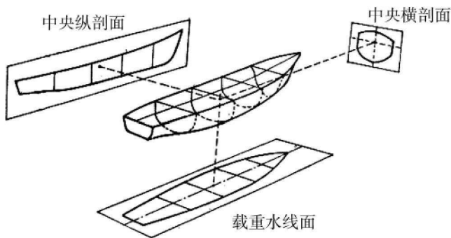
图 1-1-12 船体 3 个互相垂直剖面的投影
