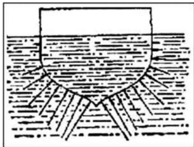
图1-1-1 船体水下部分单位面积 水压力的分布情况
