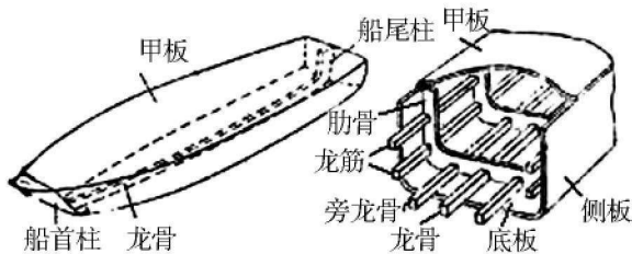
图 1-1-4 舰船模型船体的结构
