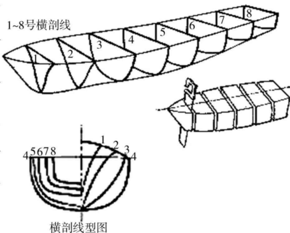
图 1-1-14 横剖面与横剖面线型图
