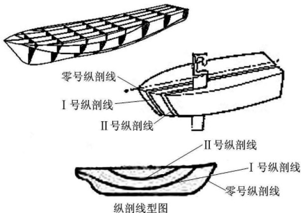
图 1-1-13 纵剖面与纵剖线型图
