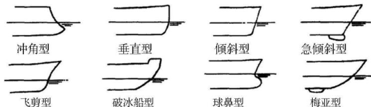
图 1-1-9 艏部形状
