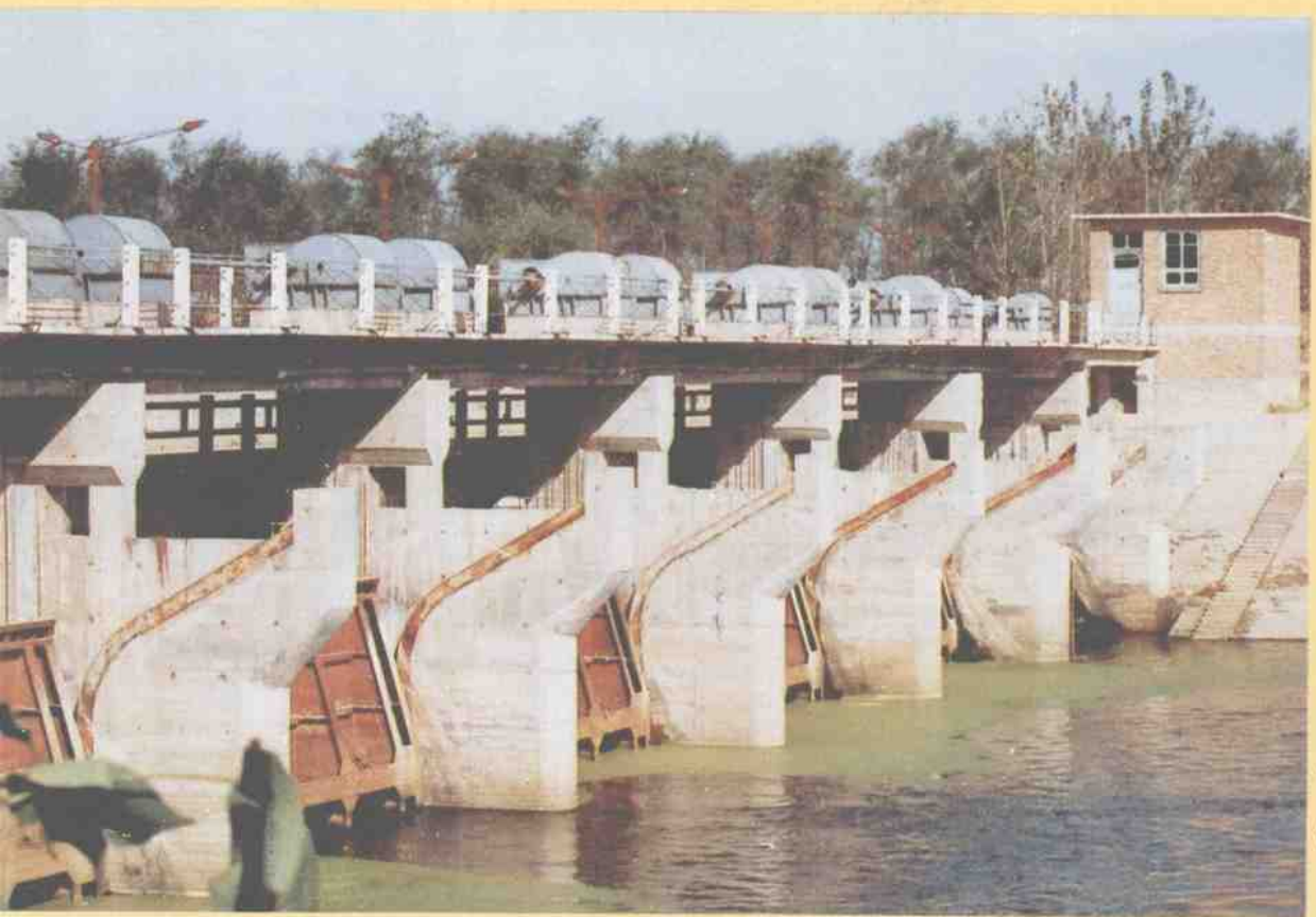
挽庄节制闸（下游）
