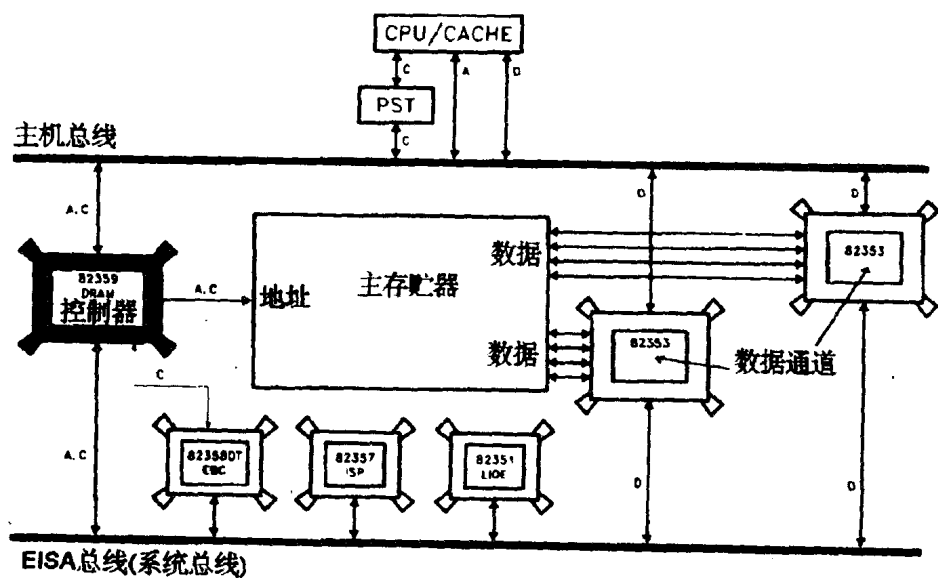
图 0-1 82359 标准配置图
