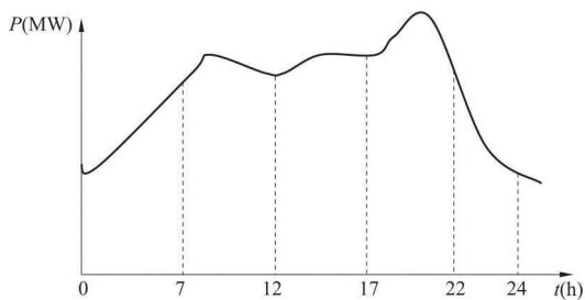
图 2-1 日用电负荷曲线
