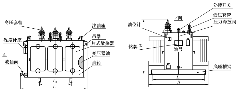
图 1-2 非晶合金铁心变压器的组成
