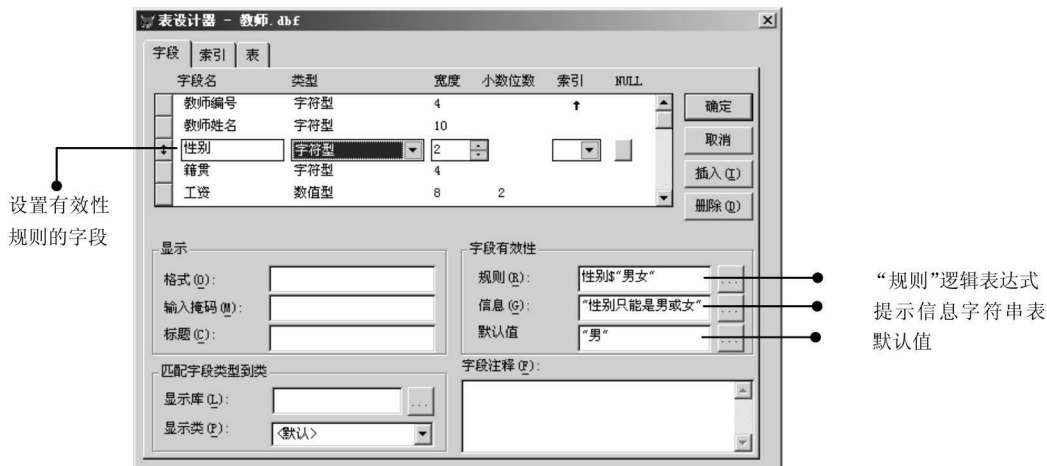
图 1-9 域完整的设置
