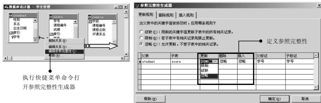
图 1-10 参照完整性设置
