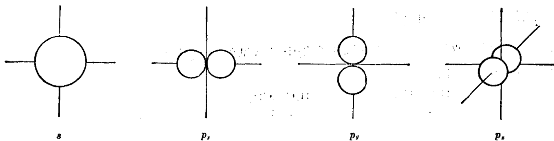
图 1-1 s 和 p 电子的轨道形状
