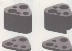
NC加工用固定块组件32mm厚度型
