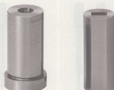
防废料回跳规格指定型凹模 肩型 直杆型
