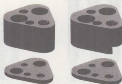
NC加工用固定块组件25mm厚度型
