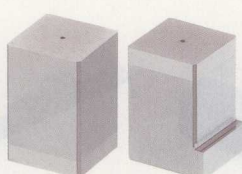
基本型方形凹模 直杆型 单边凸缘
