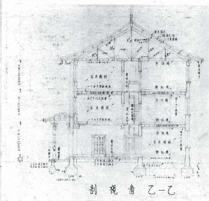
剖面图
