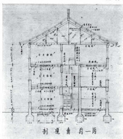
剖面图
