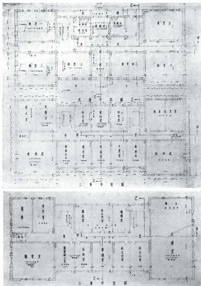
辦公廳及教室平面圖
