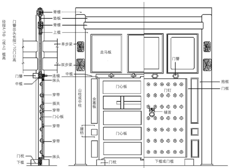
图2-1-1 《清式营造则例》棋盘门构成
