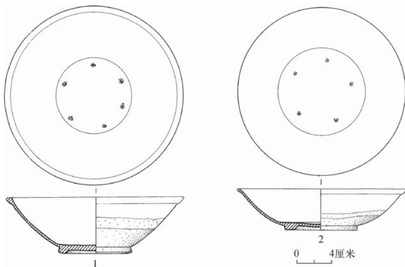
图四 M1随葬瓷碗(二)
