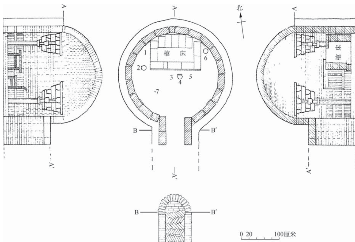
图二 M1平、剖面图
