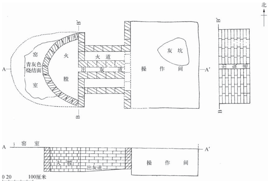
图一 京沪高铁Y1平、剖面图
