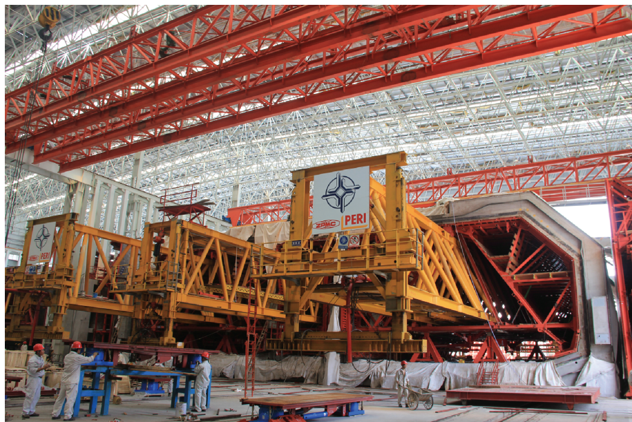
沉管管节内模
