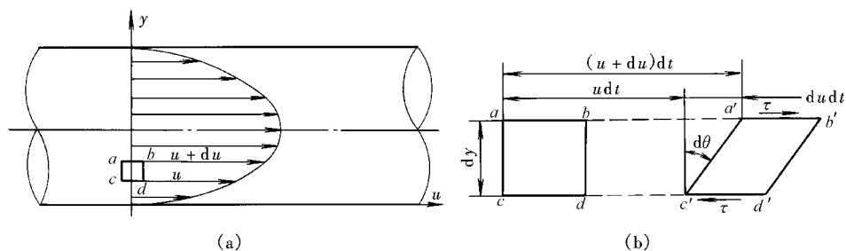
图 1-1 管内流速分布
