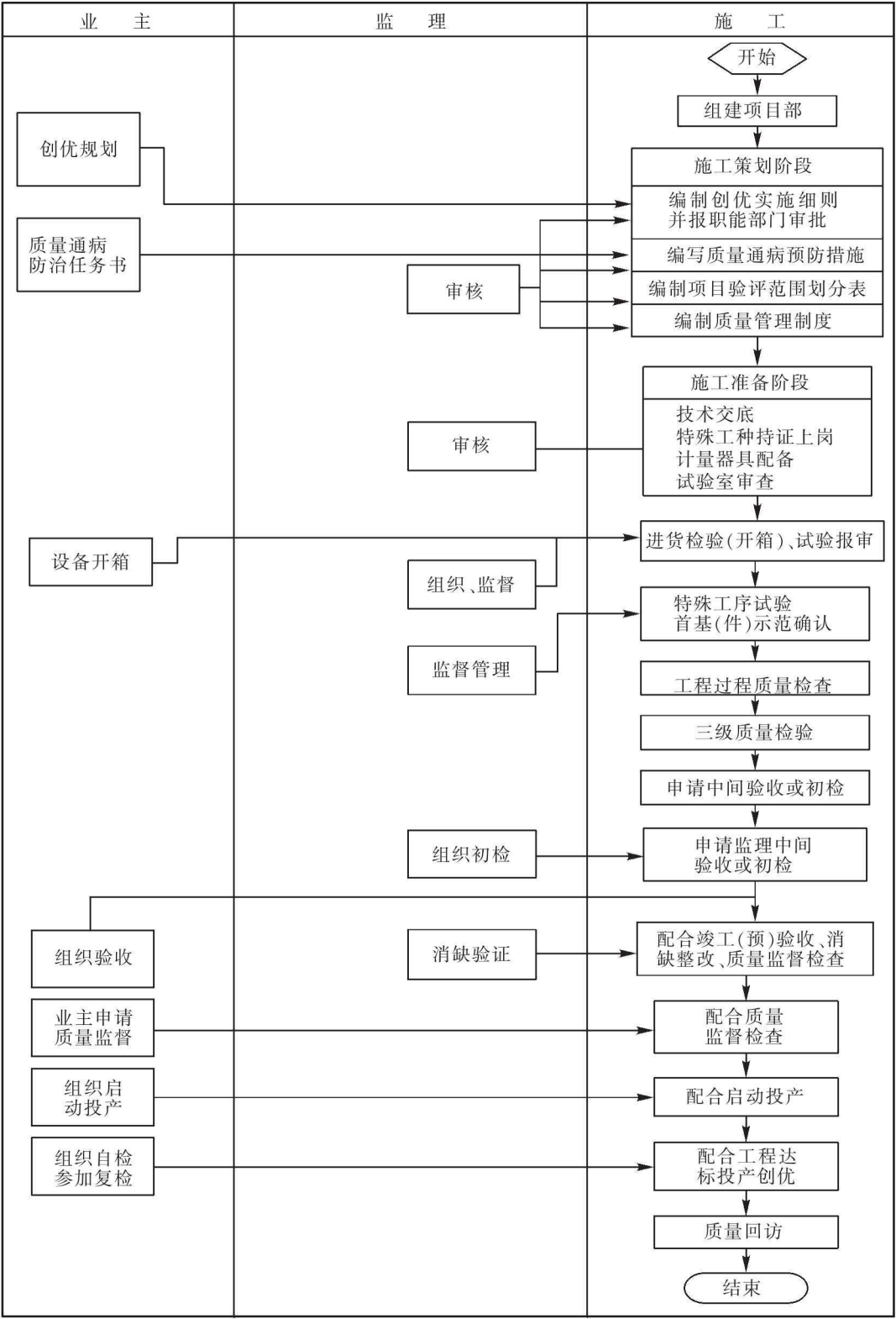
图 1-5 输变电工程质量管理的总体流程
