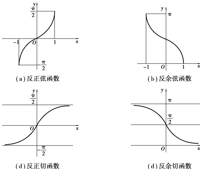
图 1.16 反三角函数图像
