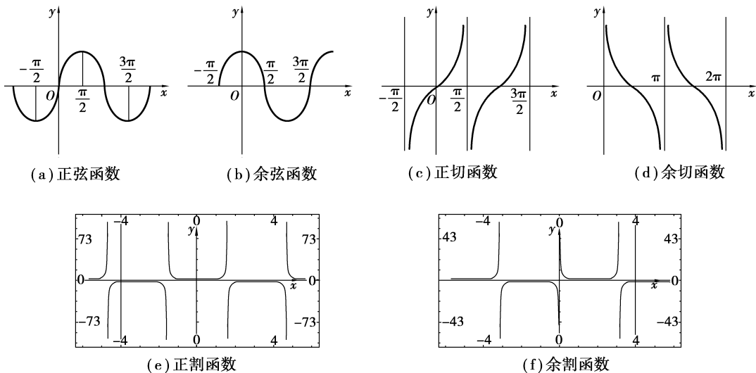
图 1.15 三角函数图像
