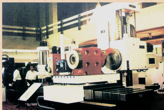
1997年，中捷友谊厂生产的我国首台数控机床
