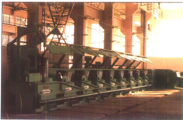
引进德国科赫公司专有技术制造的LZ9/600直线式漏渣辊拉丝机
