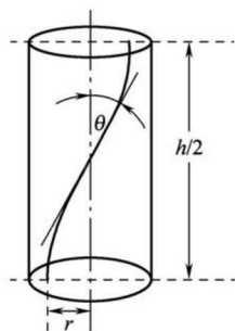
(a) 半个捻回内纤维理论几何路径
