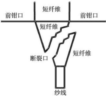
图 1.1.3 传统环锭纺细纱断头
