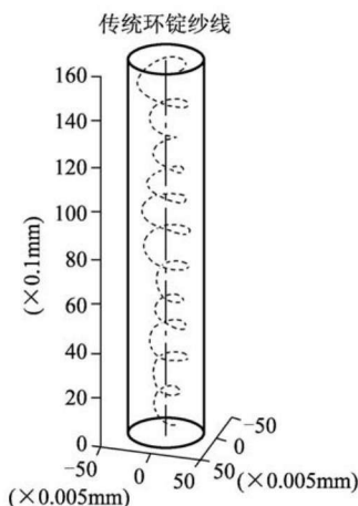
图 1.1.4 传统环锭纱线中纤维经典转移轨迹 [15]
