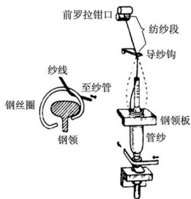
图 1.1.1 环锭纺纱的细纱加捻过程 [5]
