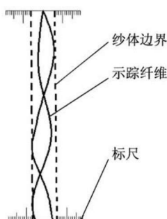
(b) 纱体内示踪纤维的转移
