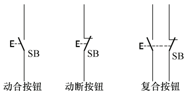
图 1-17 按钮的图形符号和文字符号
