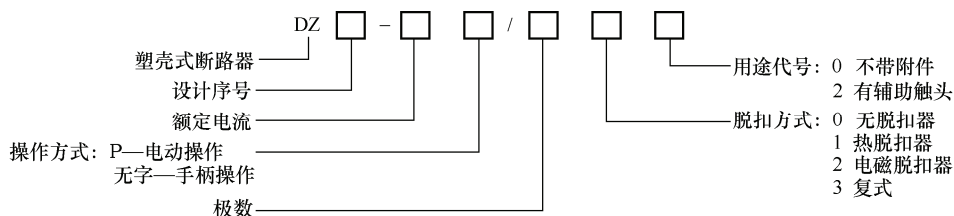
图 1-12 DZ 系列断路器的型号含义
