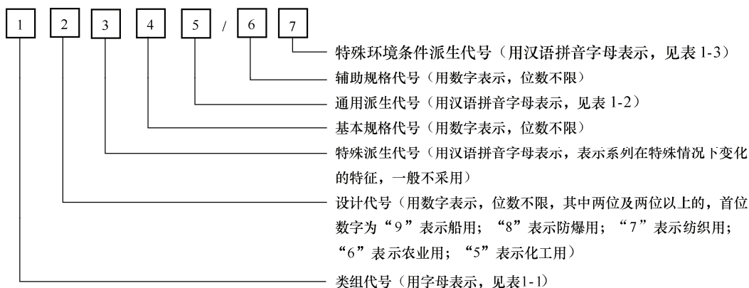
图 1-1 低压电器的型号图
