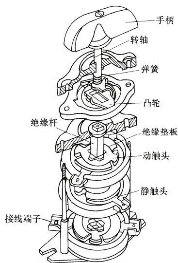
图 1-7 组合开关内部结构
