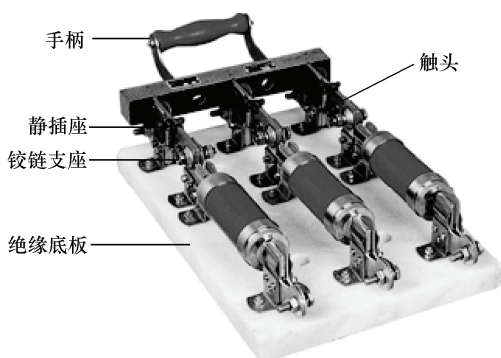
图 1-2 刀开关结构
