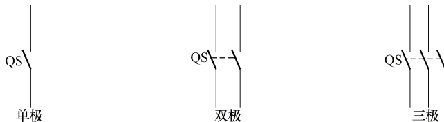
图 1-3 刀开关的图形符号
