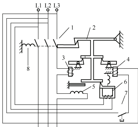
图 1-11 低压断路器的工作原理
