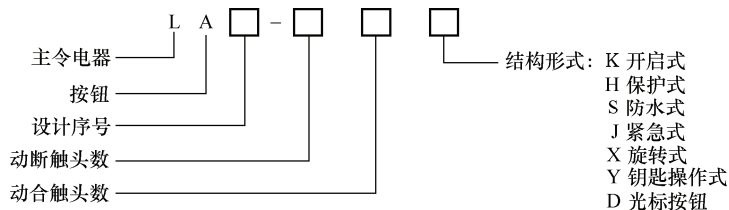
图 1-15 按钮开关的型号含义
