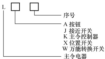
图 1-13 主令电器型号含义
