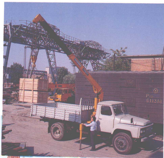
TM—30ZH 3 吨随车起重机。
