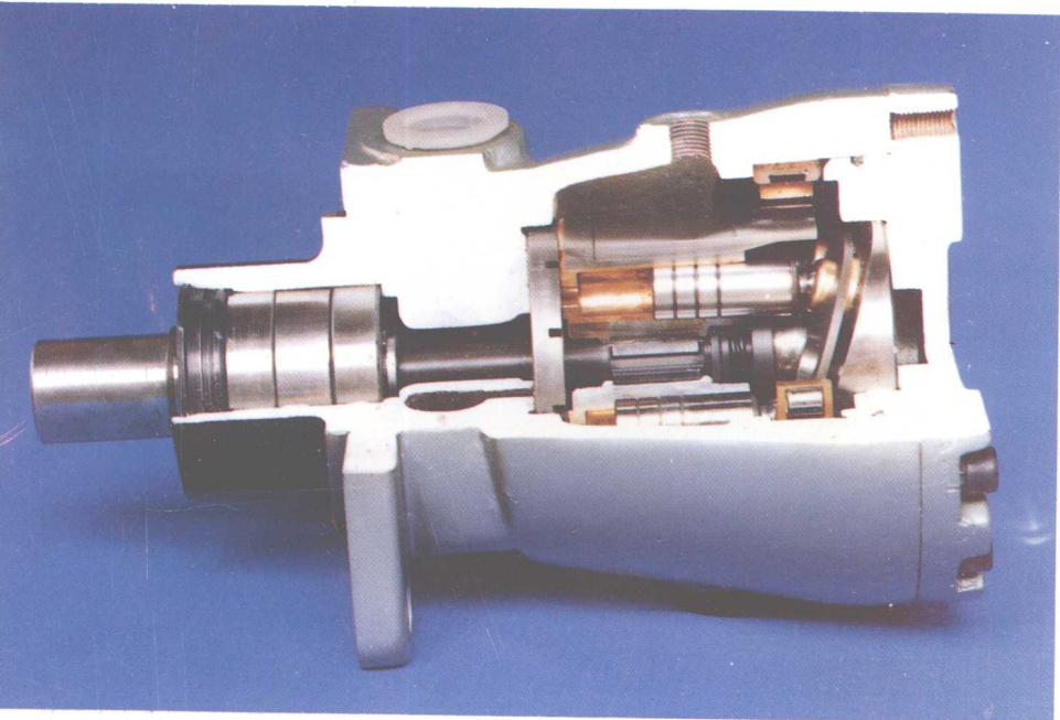
部优产品Z B D 40 轴向柱塞泵。
