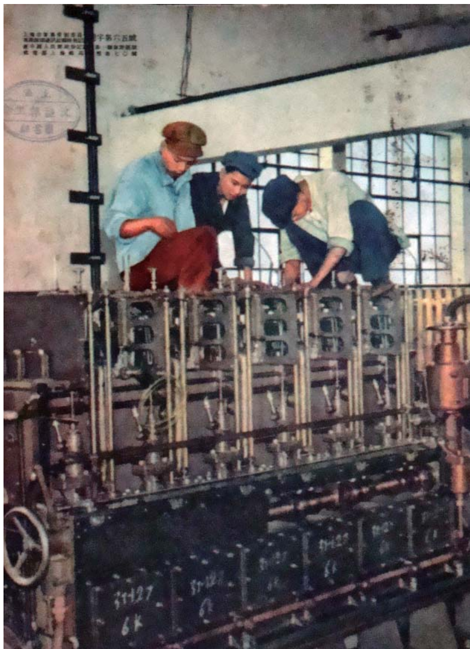
上海通用机器厂制造的第一部 300 匹马力的柴油机 (1952)
