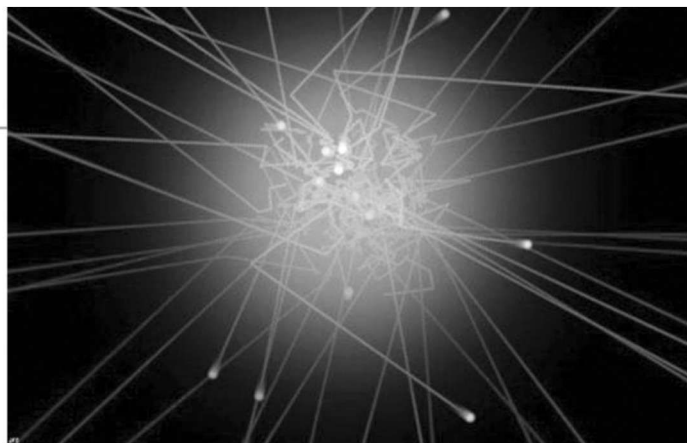
光子示意图
