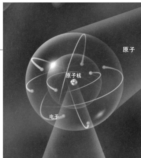
原子结构
