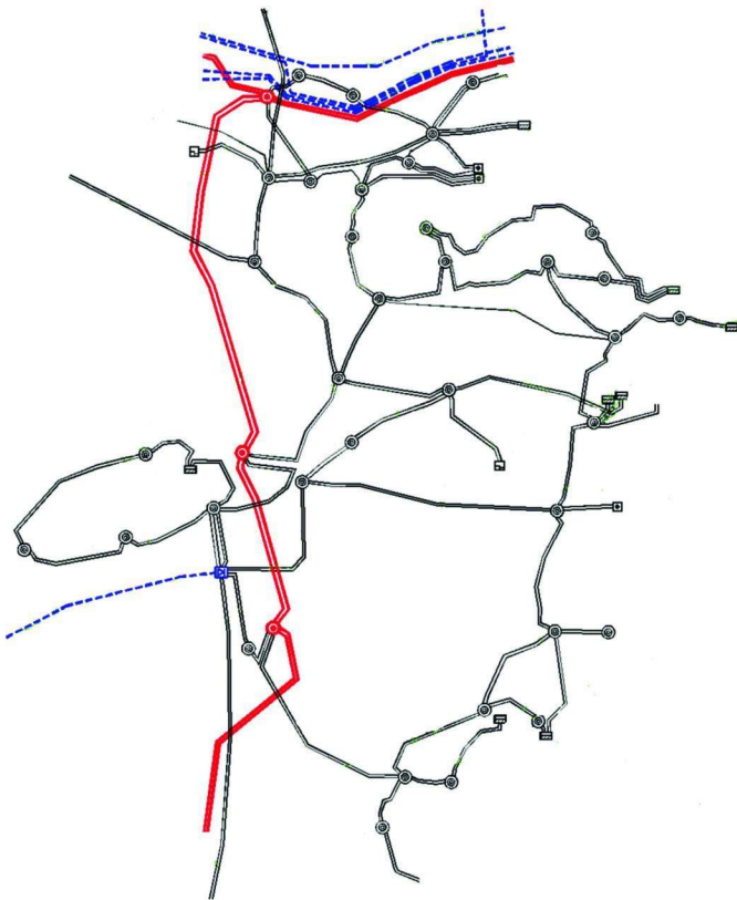
图 1-7 2014 年浙江 500 千伏及以上电网接线示意图
