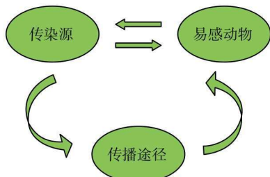
图 1-1 传染病流行示意
