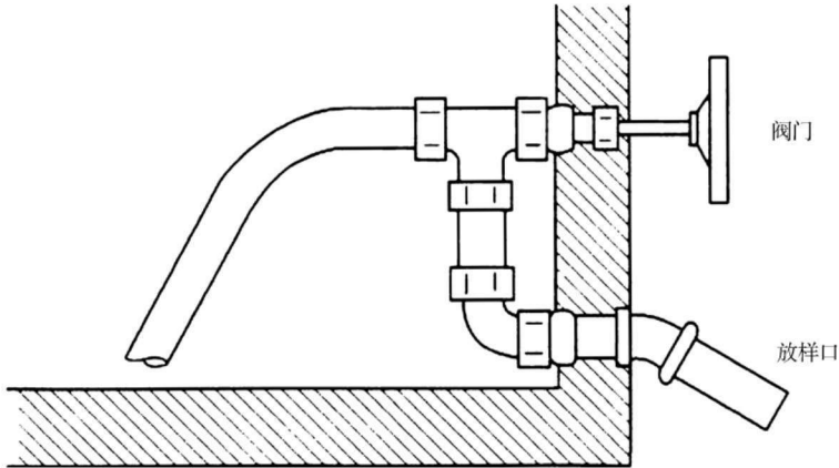
图 1-1-1 沥青取样阀
