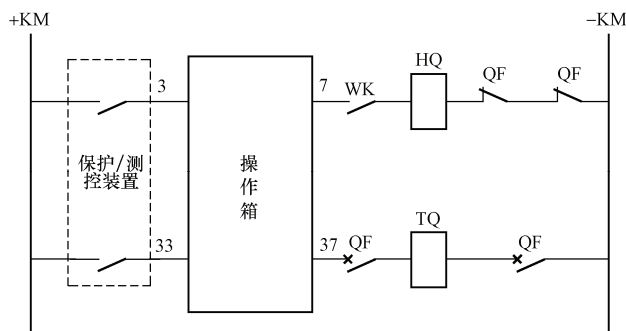
图 1-2 开关分合闸控制回路图
