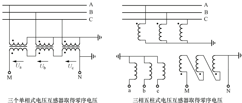
图 1-1 电压互感器取得零序电压
