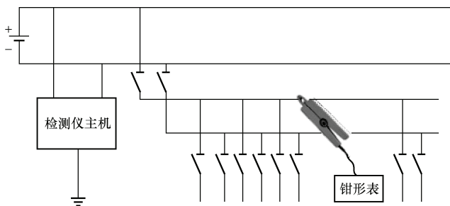
图 1-3 检测电路
