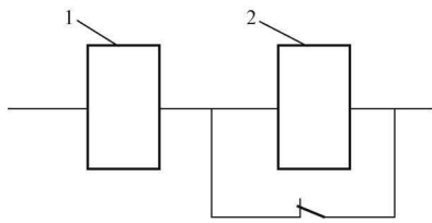
图 1-10 直流接触器双绕组线圈接线图
