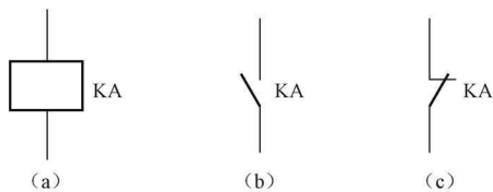
图 1-12 电磁式继电器图形、文字符号
