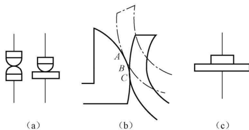
图 1-4 触头结构形式图
