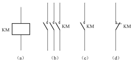
图 1-8 接触器的图形、文字符号
