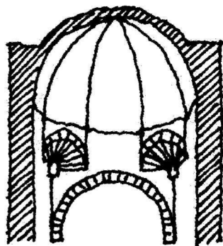
图7 抹角拱
