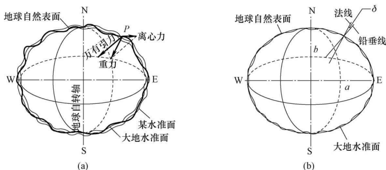
图 0-2 地球自然表面、水准面、大地水准面、参考椭球面、铅垂线、法线间的关系
