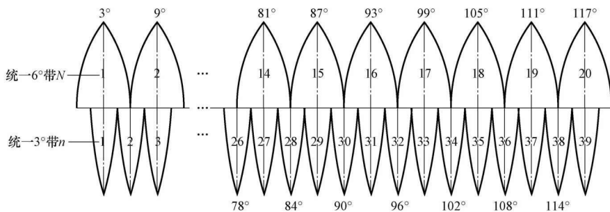
图 0-5 统一 6°带投影与统一 3°带投影高斯平面坐标系的关系
