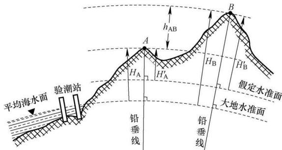
图 0-6 高程与高差的定义及其相互关系
