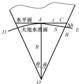
图0-7 水准面的曲率 对水平距离的影响
