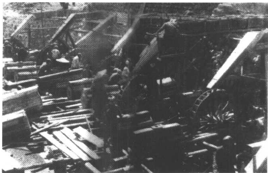
为高炉群安装水力运转风箱
