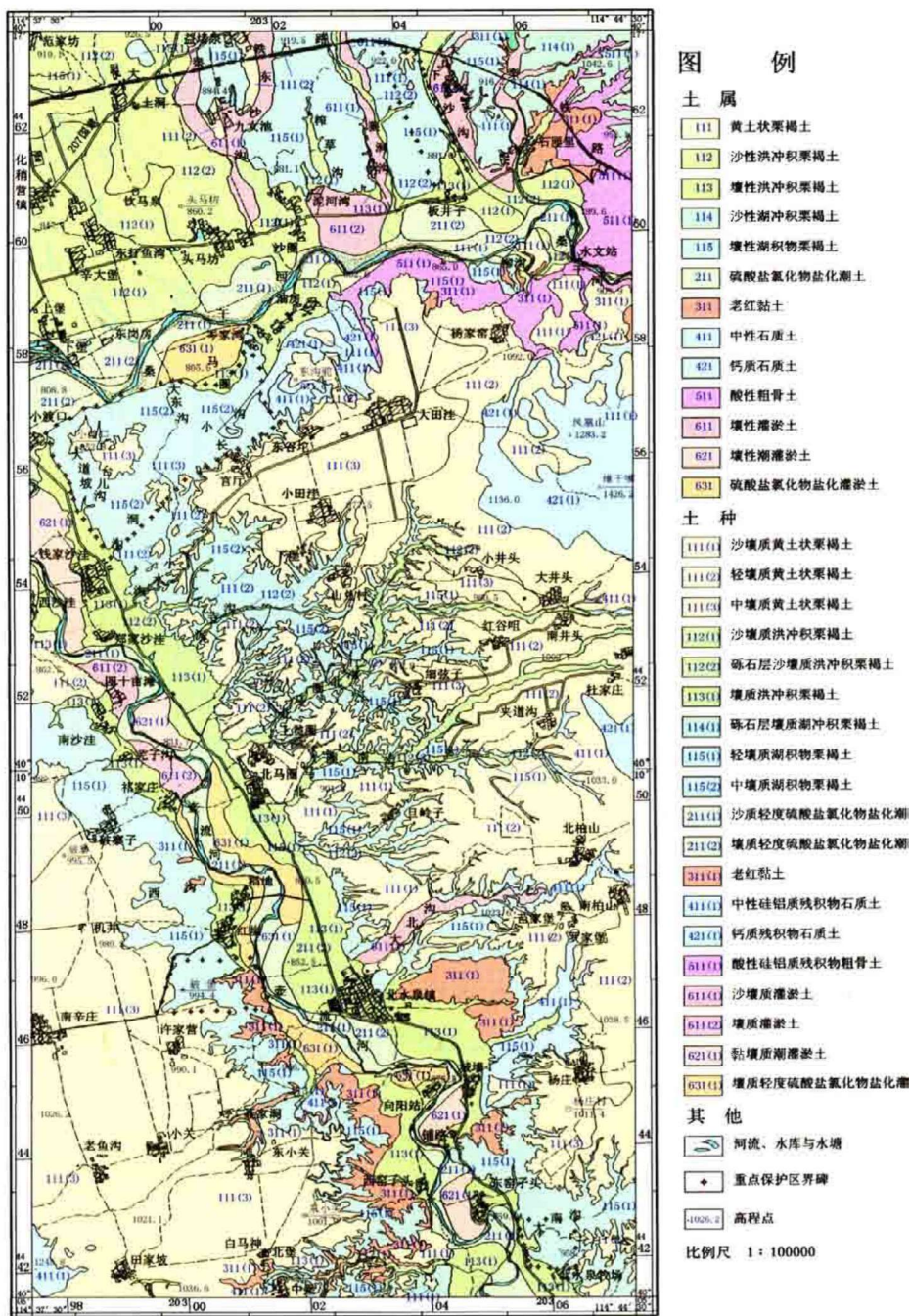
图 6 河北省泥河湾国家级自然保护区土壤图
