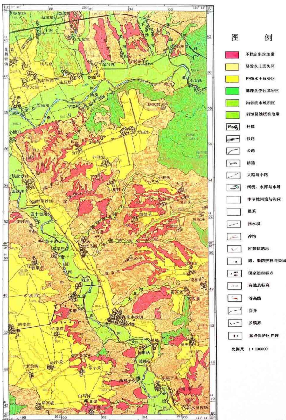
图 4 河北省泥河湾国家级自然保护区环境地质图
