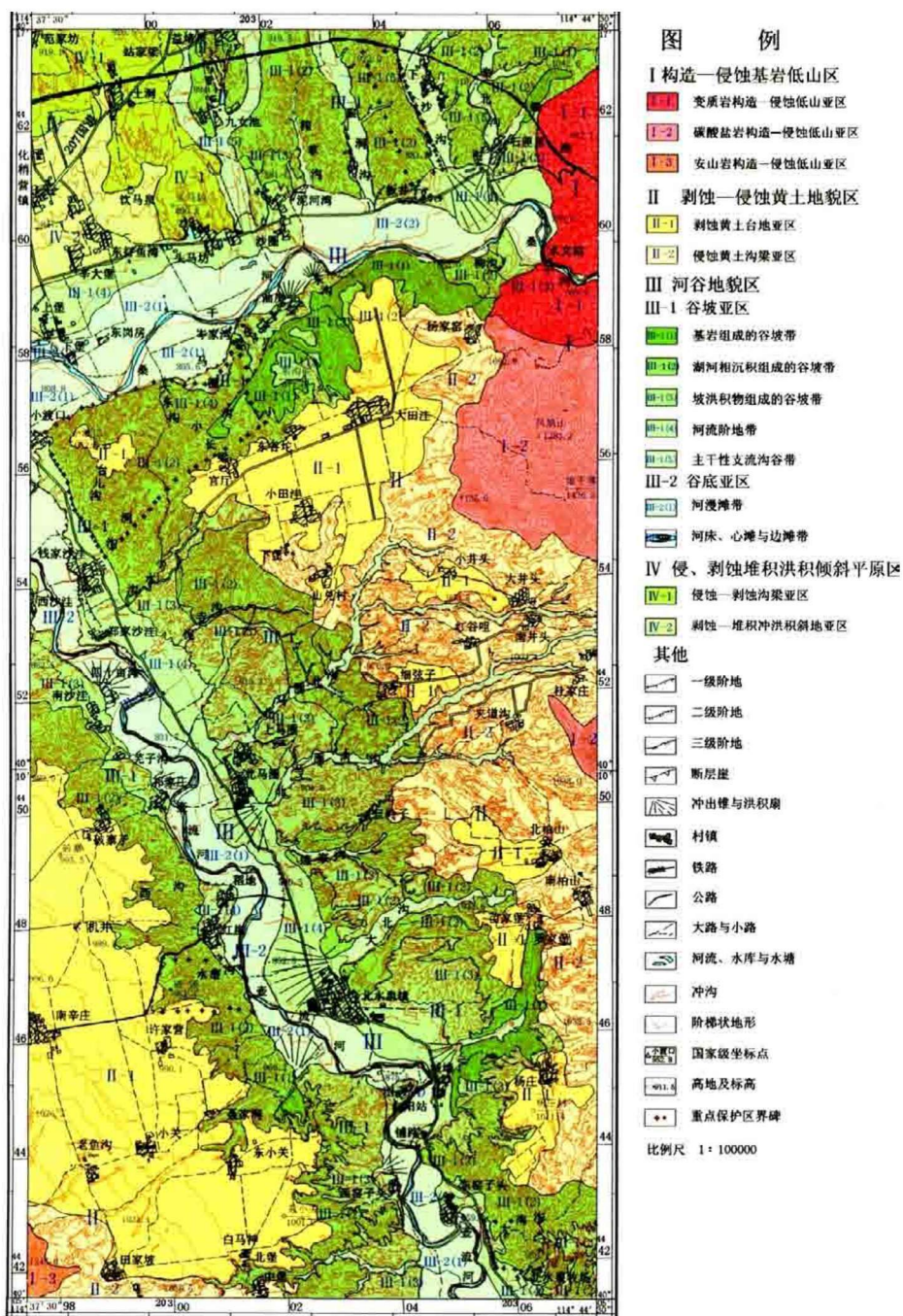
图 3 河北省泥河湾国家级自然保护区地貌图
