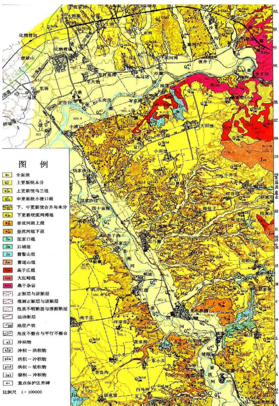
图2 河北省泥河湾国家级自然保护区地质图
