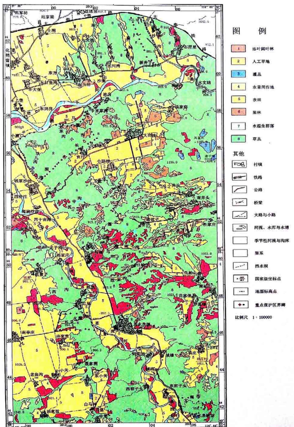
图 7 河北省泥河湾国家级自然保护区植被图
