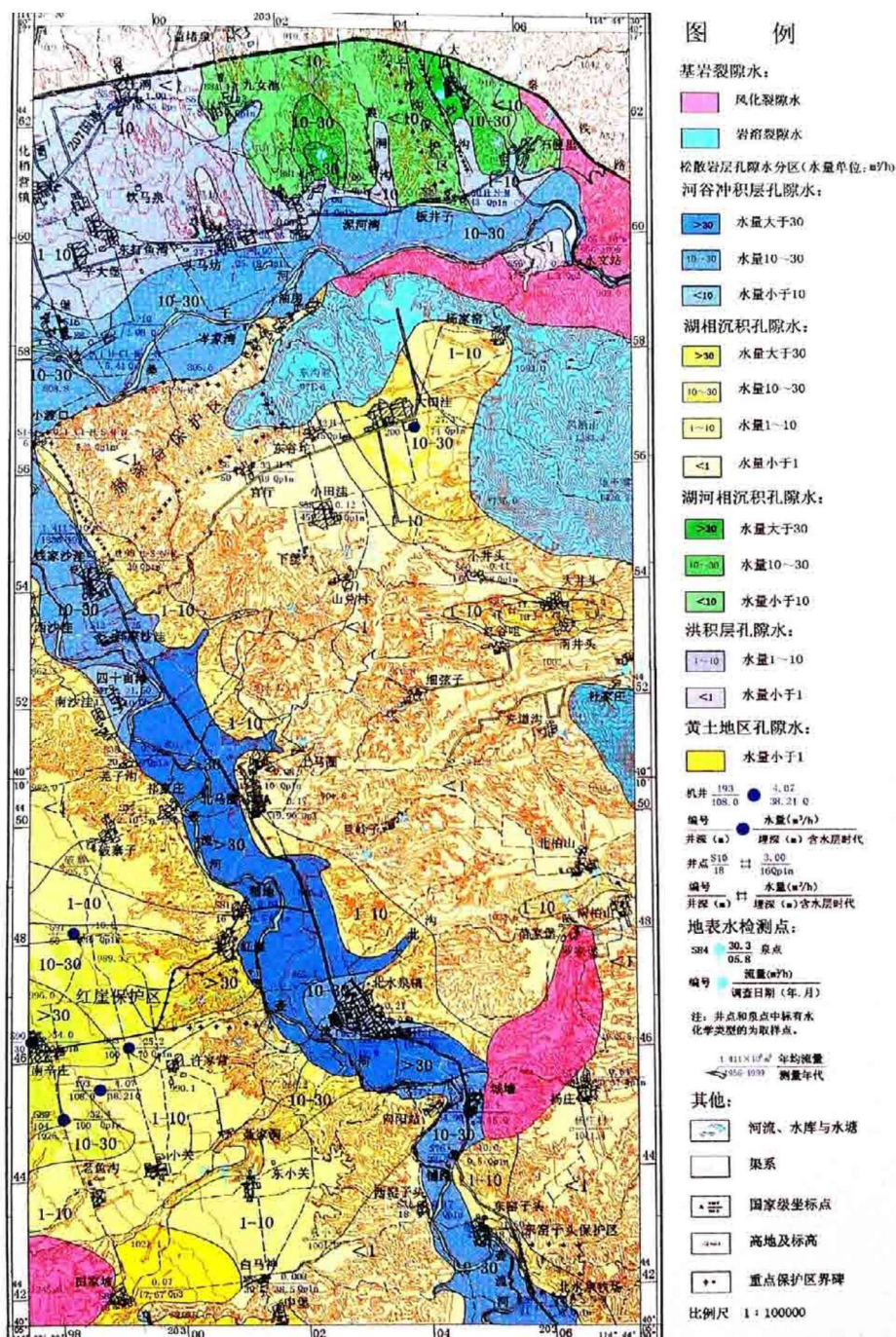
图 5 河北省泥河湾国家级自然保护区水文地质图
