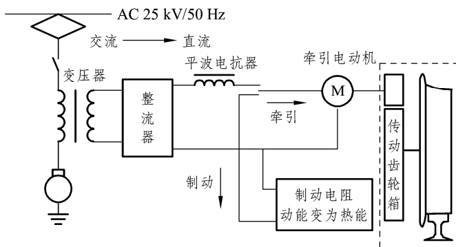
图 0.2 交-直型电力机车（EMU）的工作原理
