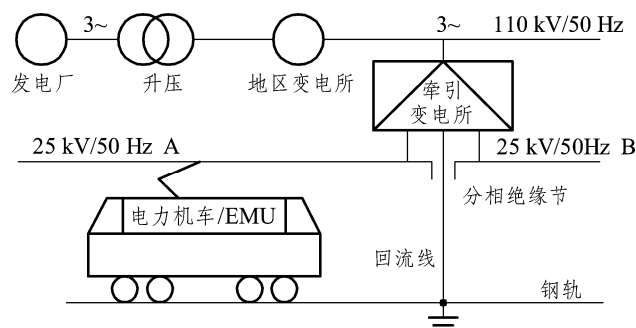
图 0.1 电气化铁道牵引供电系统结构
