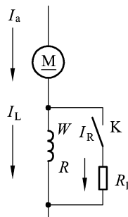
图 1.1 电阻分路法原理
