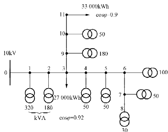
图 1-1 配电线路接线图
