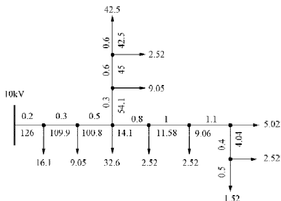
图 1-2 配电线路计算数据图
