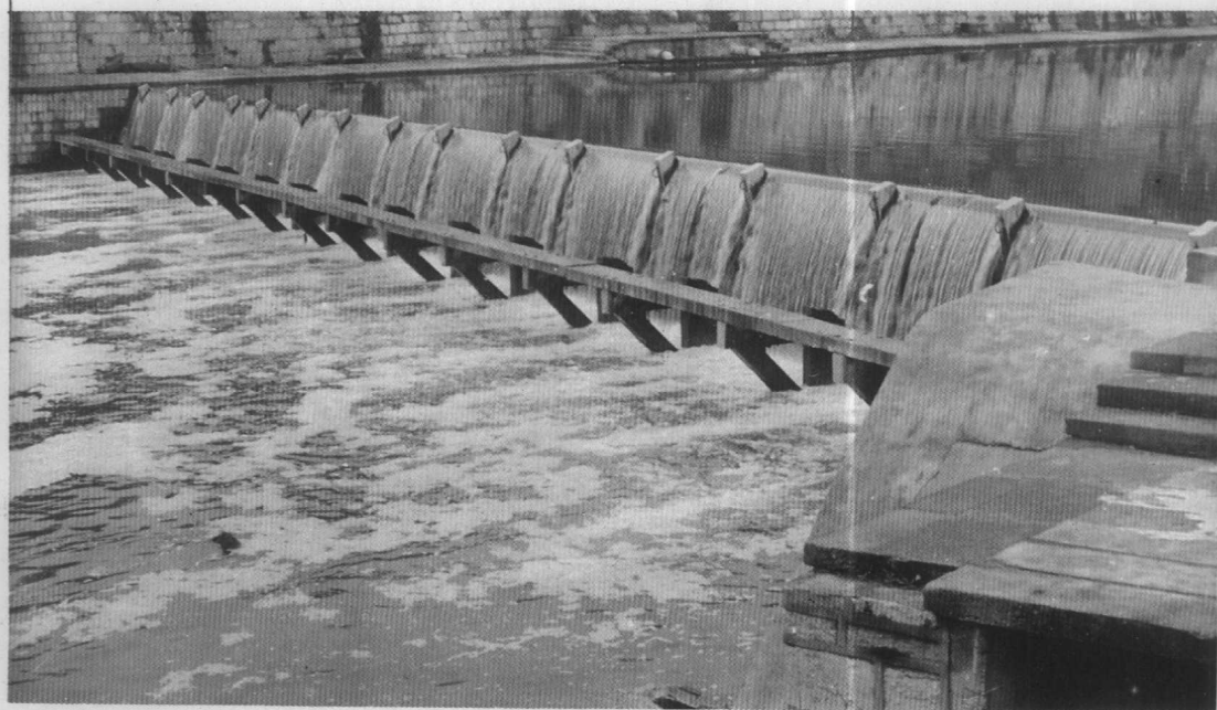
南明河翻板坝
