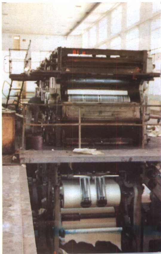
《湖北日报》社装备的铅印高速轮转机。
