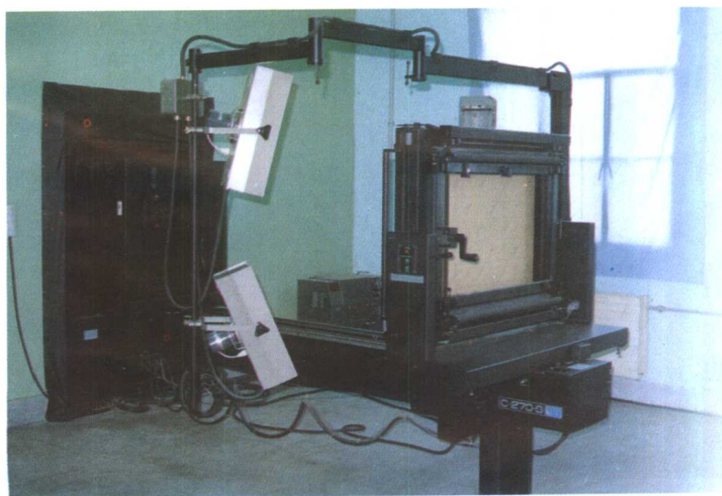
《湖北日报》社装备的现代化照相制版系统。
