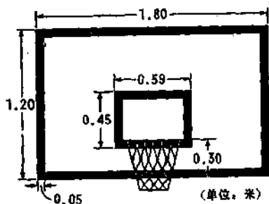
图二 篮板
