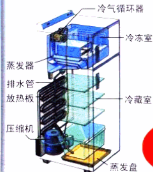
电冰箱的结构
