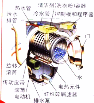
洗衣机结构
