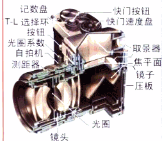
照相机的构造
